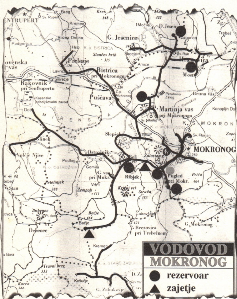
Skica mokronoškega vodovoda
