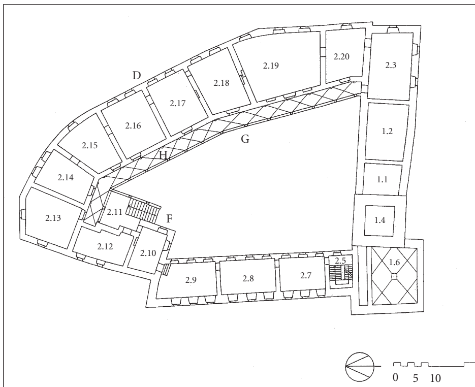
Grad Mokronog, tloris prvega nadstropja.
