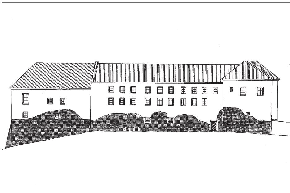
Igor Sapač, poskus rekonstrukcije podobe gradu pred letom 1943, fasada zahod s prikazom današnjega obsega razvalin.
