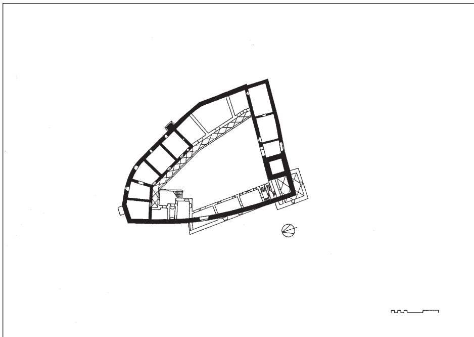
Igor Sapač, stavbni razvoj mokronoškega gradu, konec 15. stoletja.
