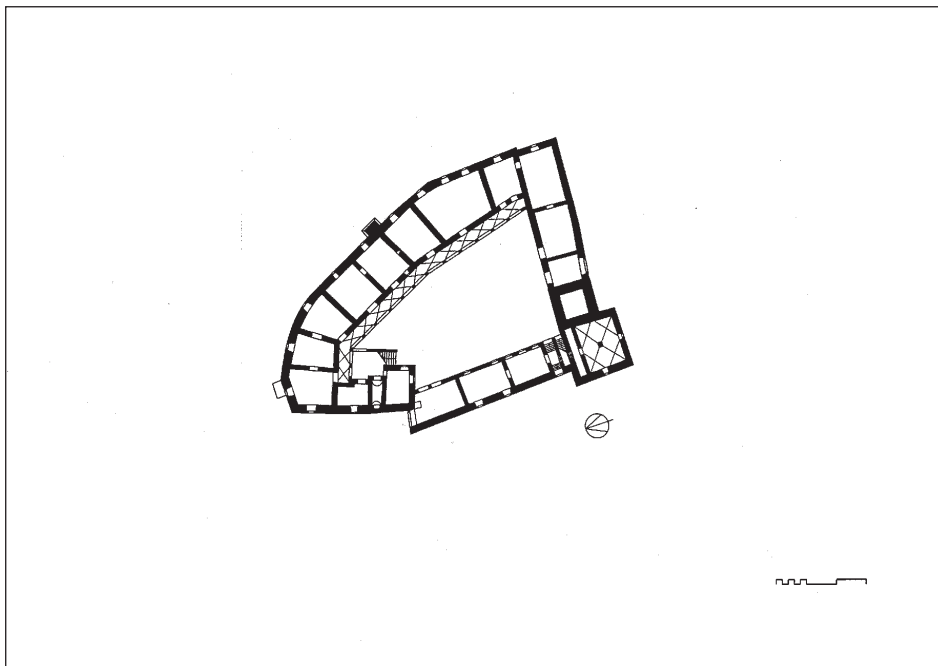
Igor Sapač, stavbni razvoj mokronoškega gradu, okoli 1770.
